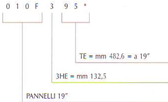
PANNELLO 19" = 482,6xHE - ALLUMINIO SPESSORE mm 3
